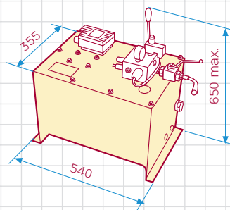
Optional Centralina con pompa a vite peso a vuoto 39 Kg (daN)
