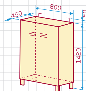
Armadio (Optional per esterno) peso a vuoto 57 Kg (daN)
