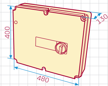
Quadro elettrico collegato alla linea 230 V - 50hz Peso 11 Kg (daN)
