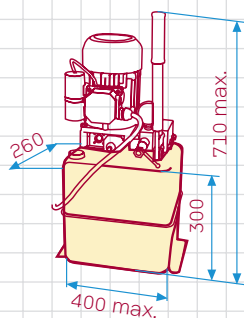
Centralina idraulica (STD) peso a vuoto 30 Kg (daN)
